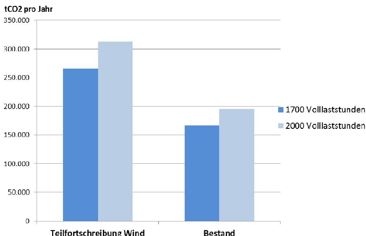
Abb. 19: CO 2 -Einsparungspotenzial der Änderung Wind bei maximaler Anlagendichte im Vergleich zum Status-quo (116,5 MW installierte Leistung) 36 für verschiedene Volllaststunden
